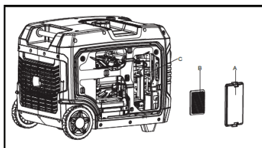
A - Couvercle du filtre à air. B - Filtre à air C - Boîtier filtre à air
